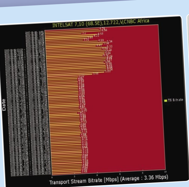
SatcoDX' scanstation bitrate meting toont hoe de CNBC Afrik transponder op 10 mei actief werd. Deze bitrate grafieken worden automatisch gegenereerd voor iedere transponder en zijn gebaseerd op continue metingen.
